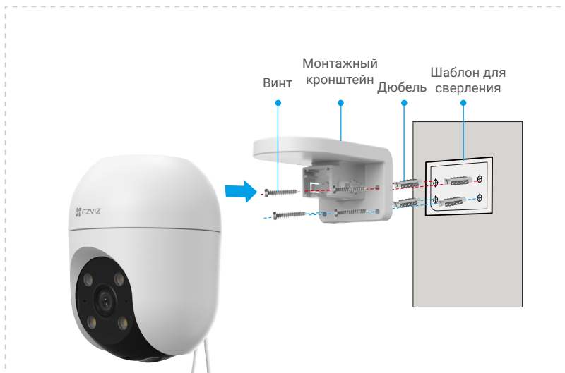
Рисунок 2. Монтаж на стену
