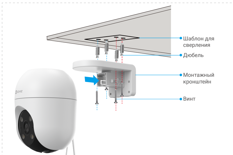
Рисунок 1. Монтаж на потолок
